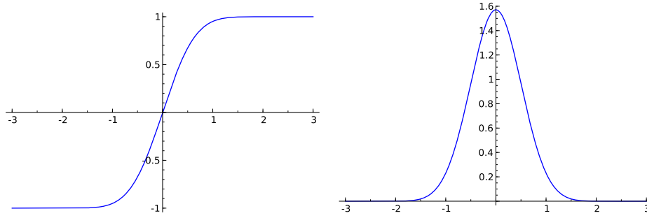
FIG. 6.3 – La transformation \varphi(t) = \tanh(\frac{\pi}{2} \sinh t) utilisée dans la méthode doublement exponentielle (à gauche) et la décroissance de \varphi'(x) (à droite).
