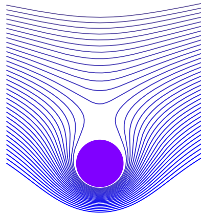
(D) Cas \alpha = 1.25 .
