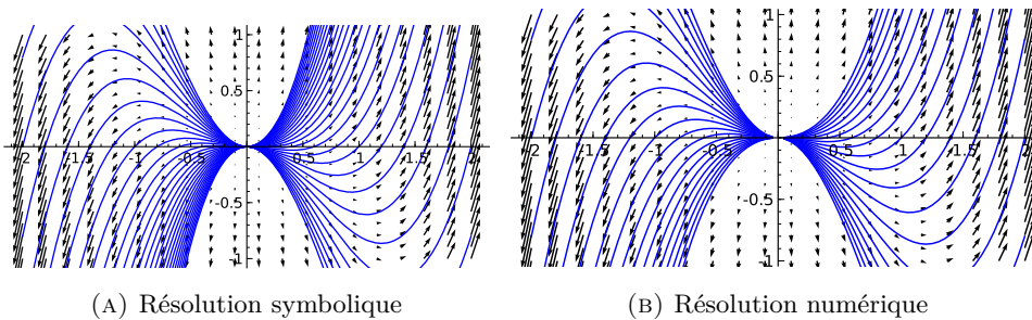
FIG. 4.10 – Tracé des courbes intégrales de xy' - 2y = x^3 .
